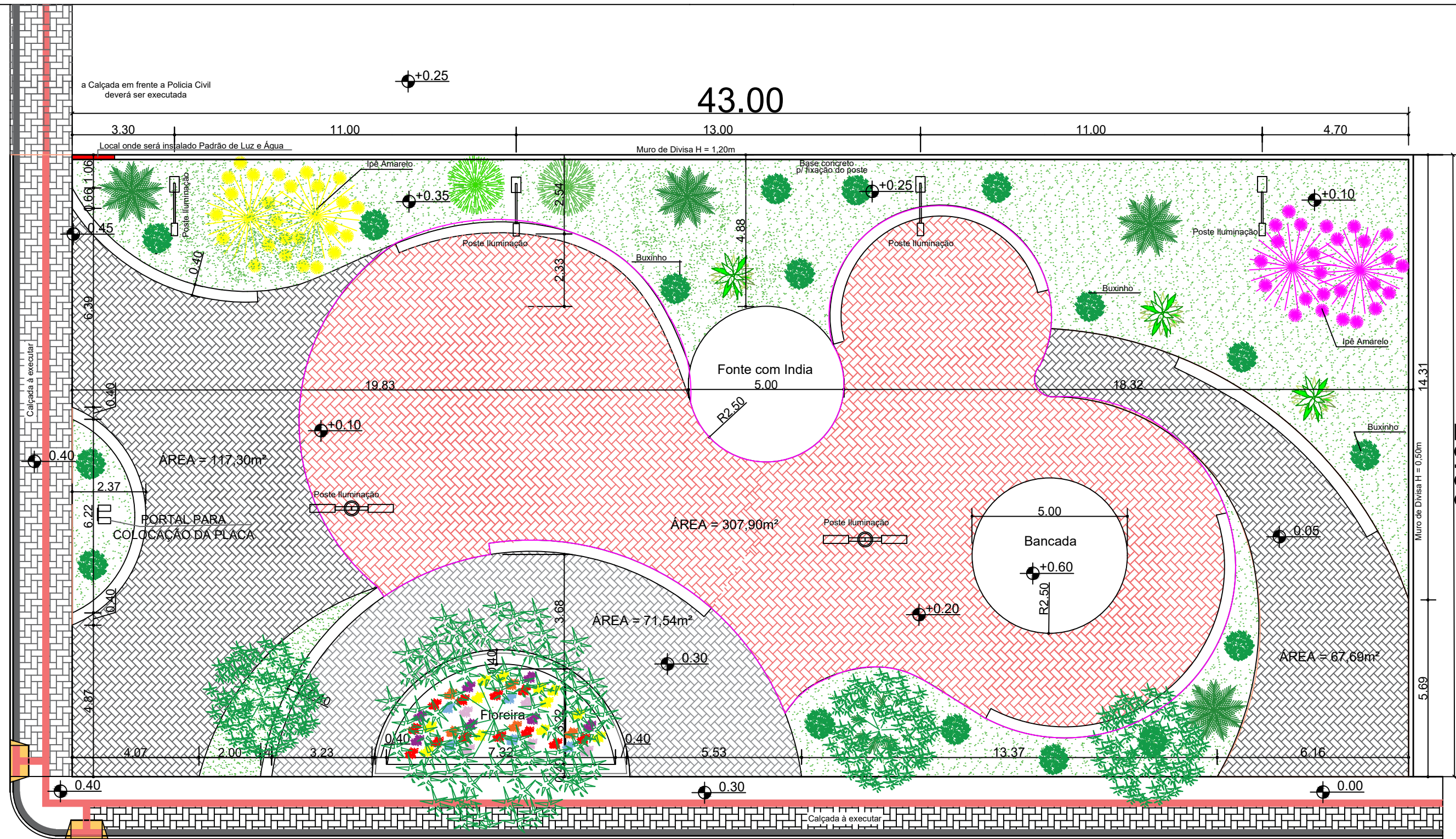
PLANTA BAIXA PRAÇA ESCALA - 1 / 75
