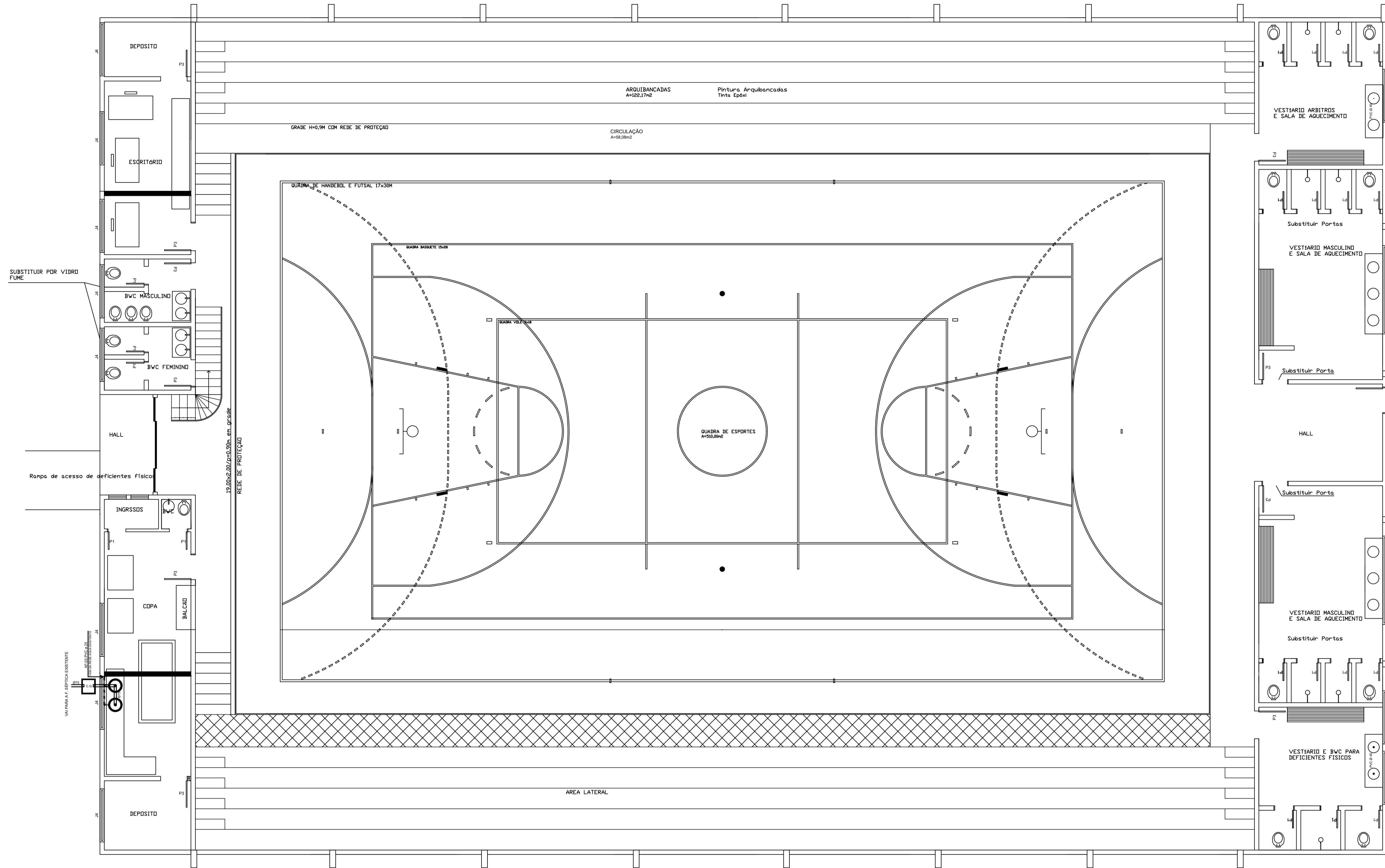
Esquema Hidro-Sanitário Pavto Térreo Escala 1/75
