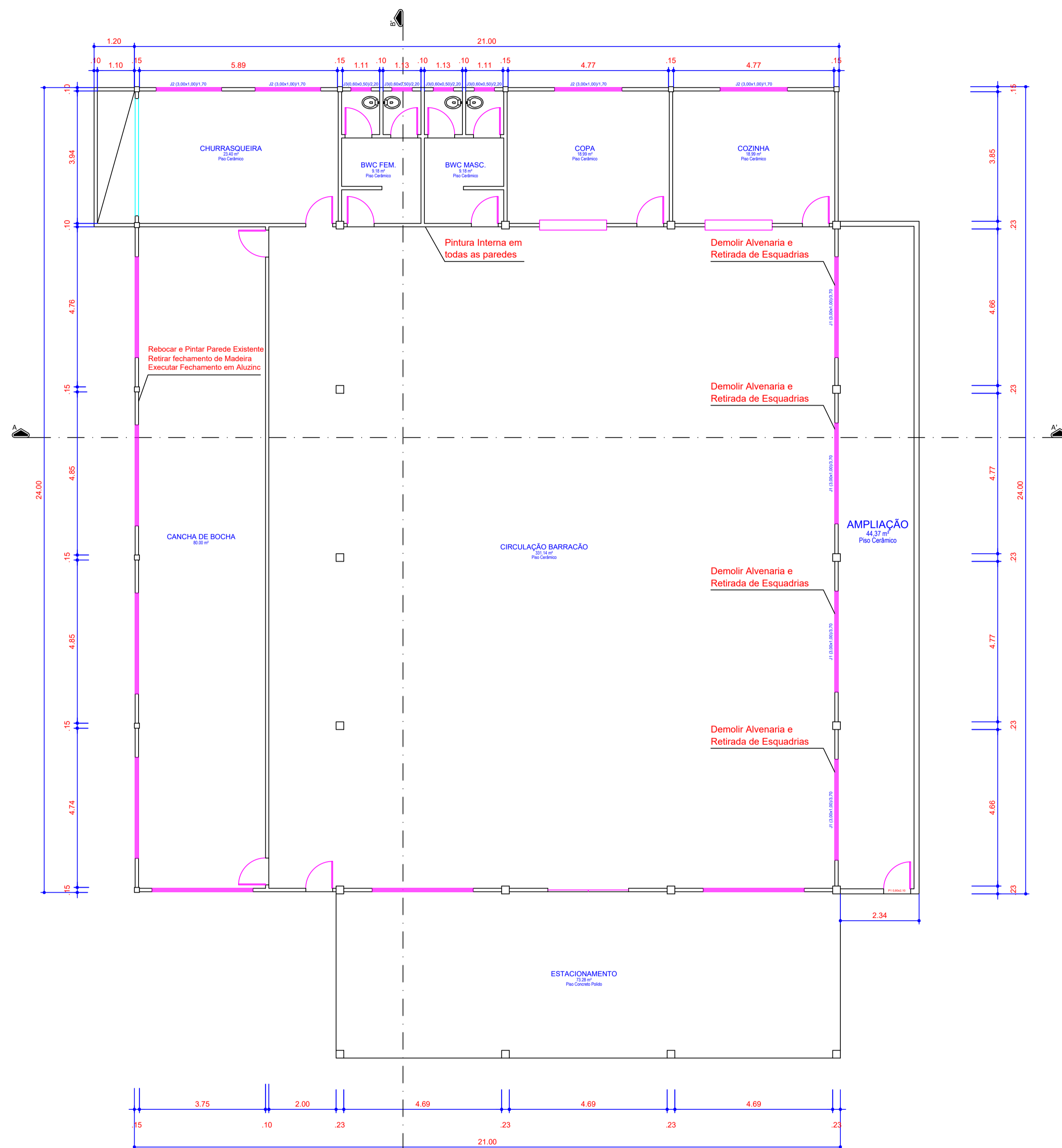
PLANTA BAIXA Área: 444,00 m² Ampliação: 46,80 m² Escala: 1/10
