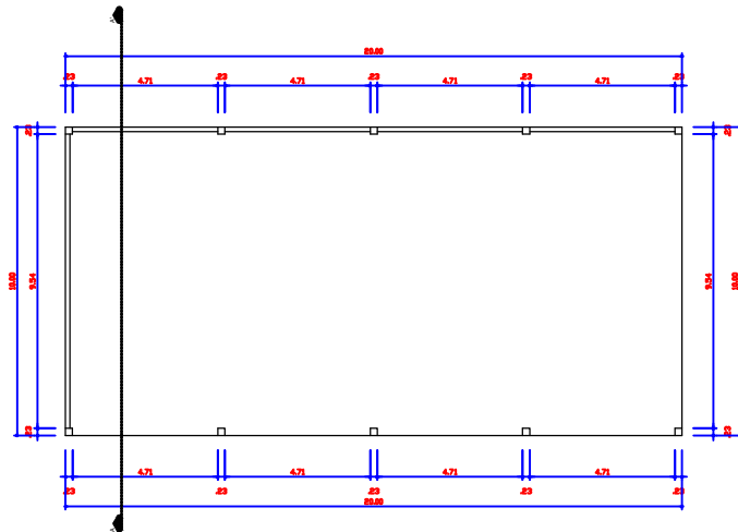
PLANTA BAIXA Área: 200,00m 2 Escala: 1/100
